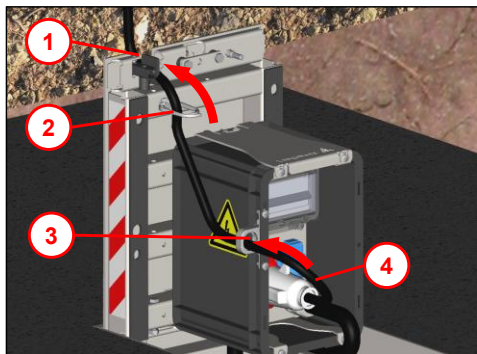
Obr. 15 Příklad vestavby elektrických komponentů
